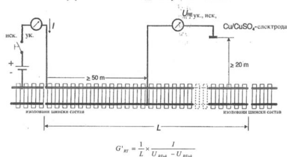
Slika 5.3. Određivanje podužne odvodnosti G'_{RE} kolosijeka na otvorenom
